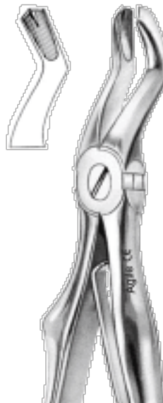
AGI-01-285 Fig. 3 upper molars obere Molaren molaires supérieures molares superiores Для верхніх молярів
